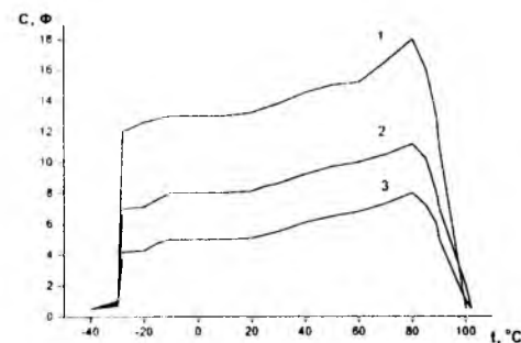
Рис.1 Температурна залежність ємності конденсаторів типорозміру "2525", електроди яких виготовлено на основі нанопористого вуглецю, отриманого з:
