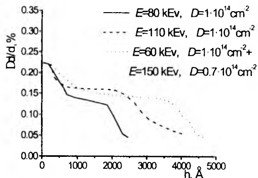
Рис. 1. Профілі деформації в ФГП, імплантованих іонами В + у режимі E=80keV, D=1*10 14 см -2 ; E=110keV, D=1*10 14 см -2 та E=60keV, D=1*10 14 см -2 + E=150keV, D=0,7*10 14 см -2 .
