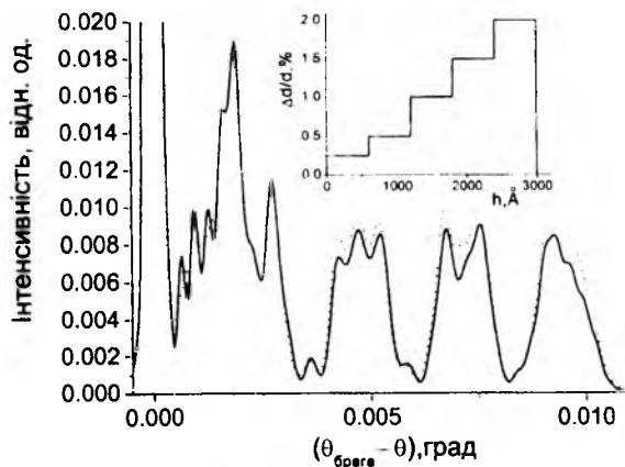
Рис. 1. Криві дифракційного відбивання, обчислені для профілю деформації, представленого на вставці: – динамічна теорія; – кінематична теорія без урахування поглинання.
