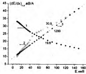
Рис. 1. Залежність енергетичних втрат, пов'язаних із пружним (1) та непружним (2) гальмуванням імплантанта та довжини проективного пробігу (3) від енергії імплантанта F^+ (ФГП складу Y_{2,8}La_{0,2}Fe_{4,54}Ga_{0,46}O_{12} ).
