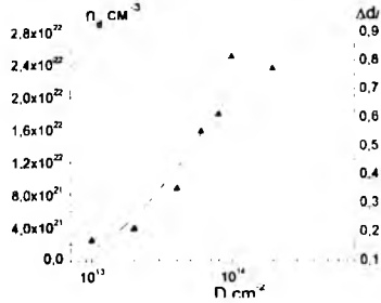
Рис. 2. Залежність відносної зміни максимальної деформації (\Delta d/d)_{\max} від дози імплантації іонами F^+ ( E=90 \text{ кеВ} ) (маркери), апроксимація рівнянням (2) (суцільна лінія) та відповідні значення концентрації зміщених атомів – пояснення в тексті
