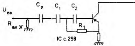
Рис. 2. Схема експрес-контролю ТПК на основі Ta 2 O 5 за рівнем другої гармоніки.
