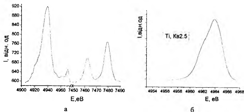
Рис. 1. Фотометрична крива рентгенівського спектра Ti від металічного порошку (а) та результат виділення Ti K_{\beta_{2.5}} (б) з інтегрального спектра.
