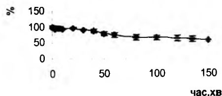
Мал.1. Вплив нагрівання ( 50^\circ C ) на активність каталази з печінки свині (n=3).
