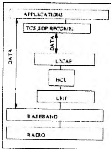
Рис.1 Стек протоколу Bluetooth.
