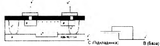
Рис.1. Тестовий елемент для визначення зарядової нестабільності міжфазної границі розподілу Si-SiO 2 .
