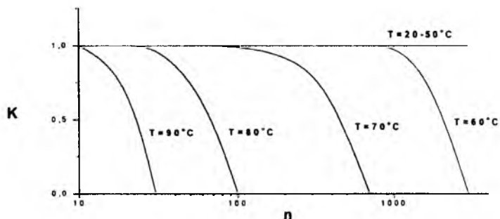
Рис. 2. Залежність кулонівської ефективності суперконденсаторів типорозміру "2525" від кількості циклів для різних температур.
